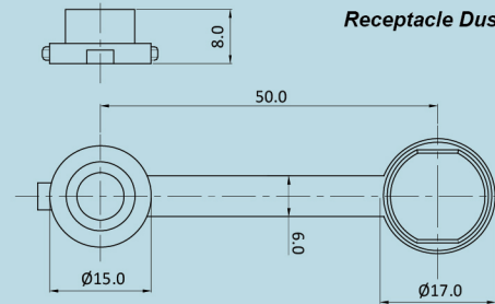
Receptacle Dust-Proof Cap
